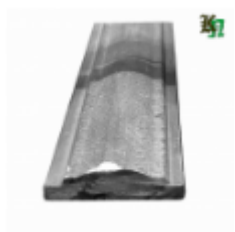
Поручень, арт. 12.083 3000x49x13мм Вес: 11 кг Цена (за шт): 3 000 руб.
