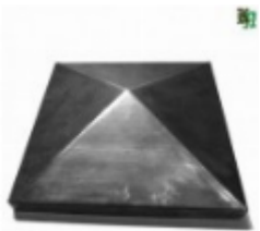
Заглушка на столб 120x120, арт. 15.058.02 120x120x1мм Вес: 0.142 кг Цена: 70 руб.
