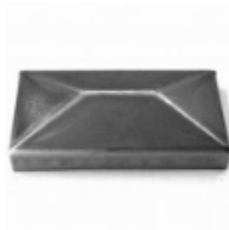
Заглушка, арт. 3060.01 30x60x1мм Вес: 0.027 кг нет в наличии
