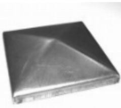
Заглушка, арт. 15.058 120x120x1мм Вес: 0.174 кг Цена: 78 руб.
