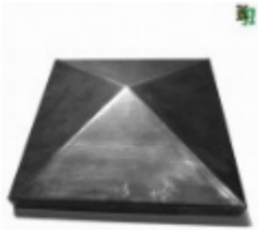
Заглушка на столб 80x80, арт. 15.056.02 80x80x1мм Вес: 0.079 кг Цена: 21 руб.
