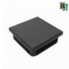
Заглушка пластиковая, арт. 35.100 кв.100x100мм Вес: 0.06 кг Цена: 45 руб.
